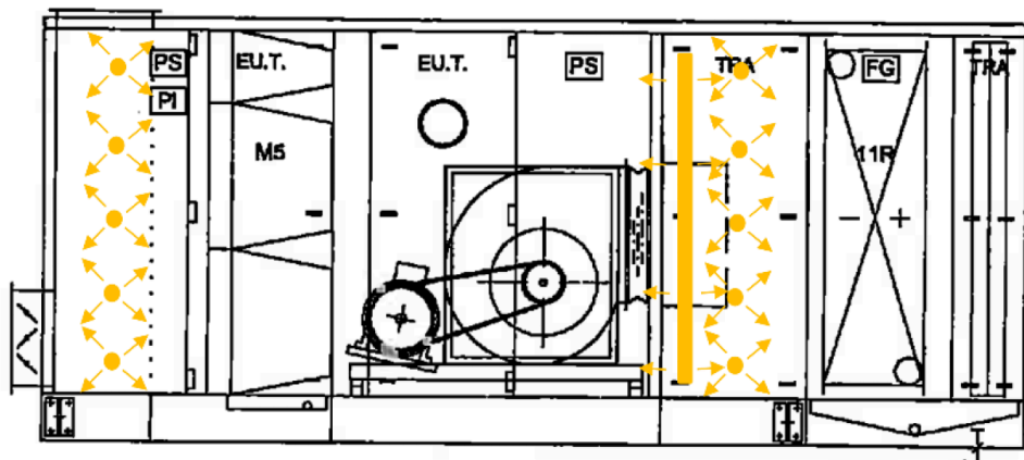
Intérieur de l'unité de traitement d'air
